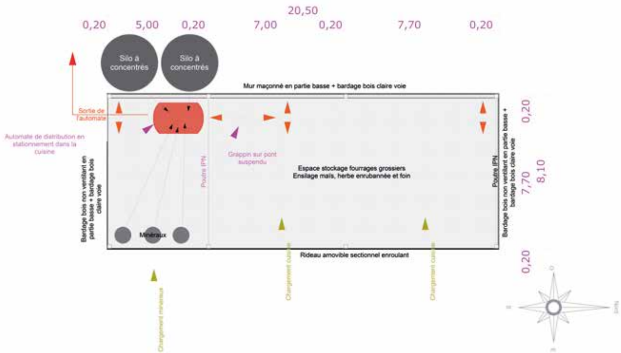
Plan 6.3 : Exemple d'aménagement interne d'une cuisine Lely (Famille B)
