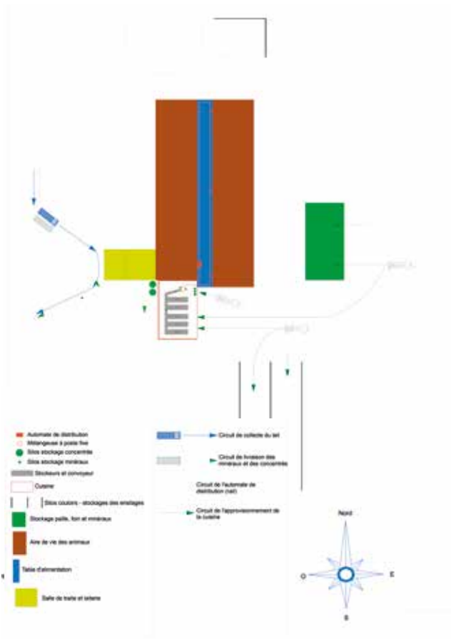
Plan 6.2 : Exemple de cuisine juxtant en pignon le logement des animaux avec un automate de distribution sur rail
