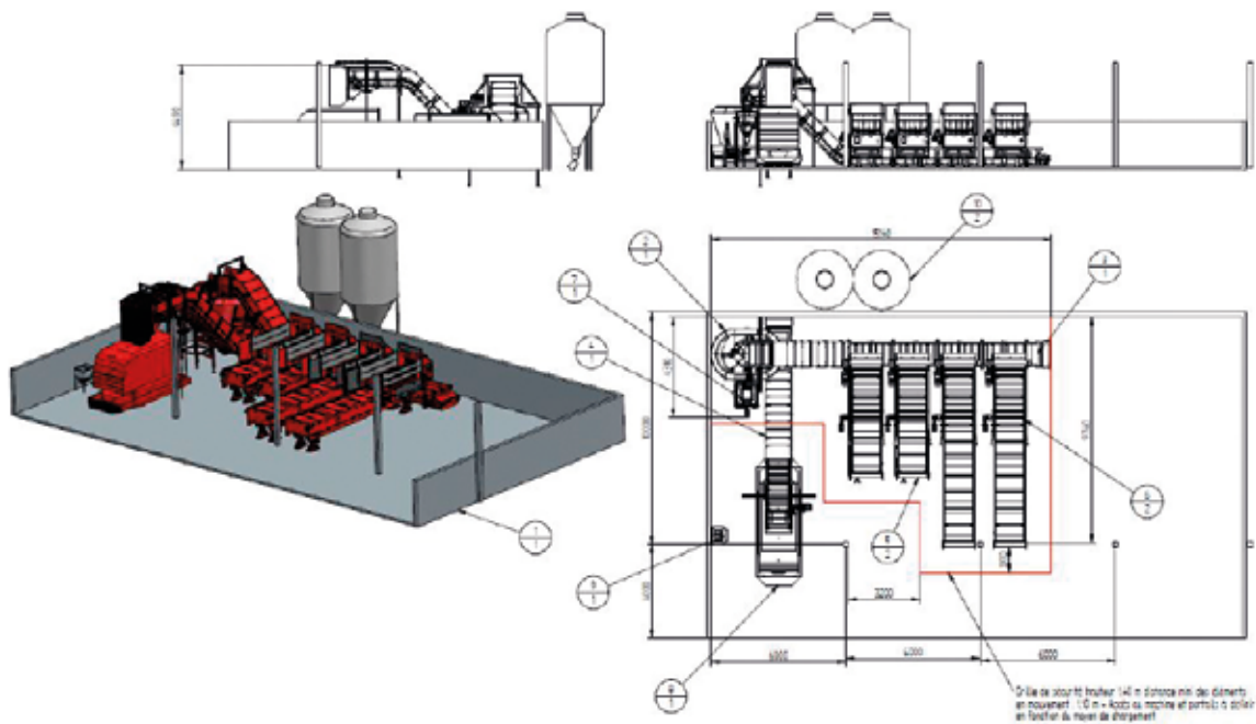
Plan 6.6 : Exemple d'aménagement d'une cuisine Jeantil (Famille D) - Source Jeantil
