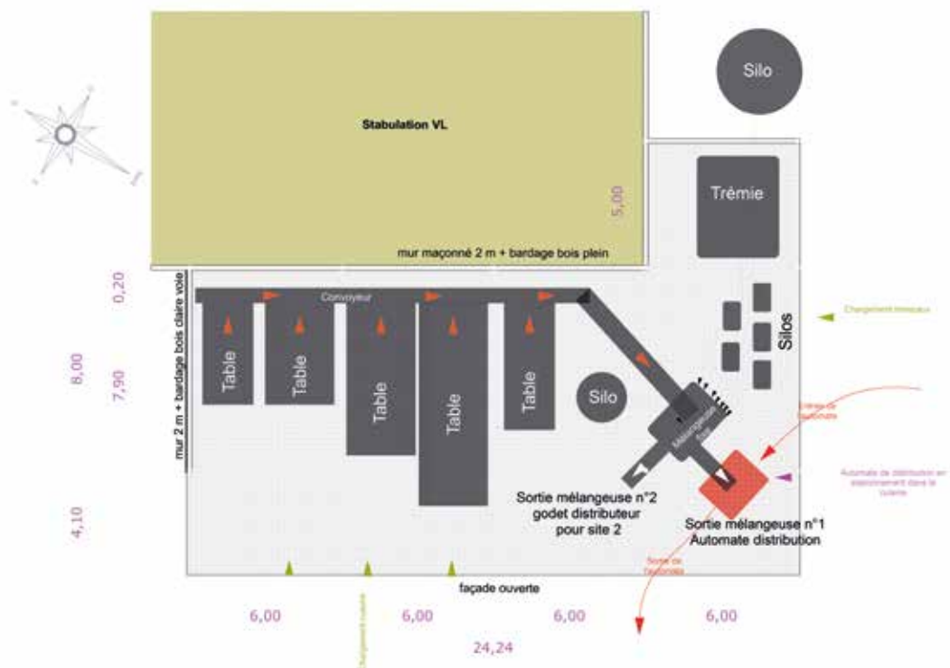
Plan 6.4 : Exemple d'aménagement interne d'une cuisine DeLaval (Famille D)
