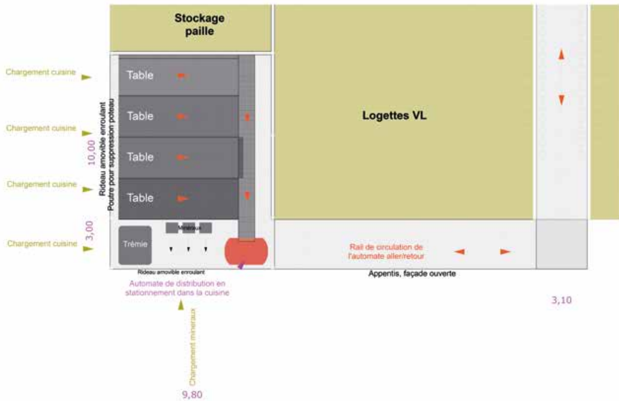
Plan 6.5 : Exemple d'aménagement interne d'une cuisine Trioliet (Famille A)
